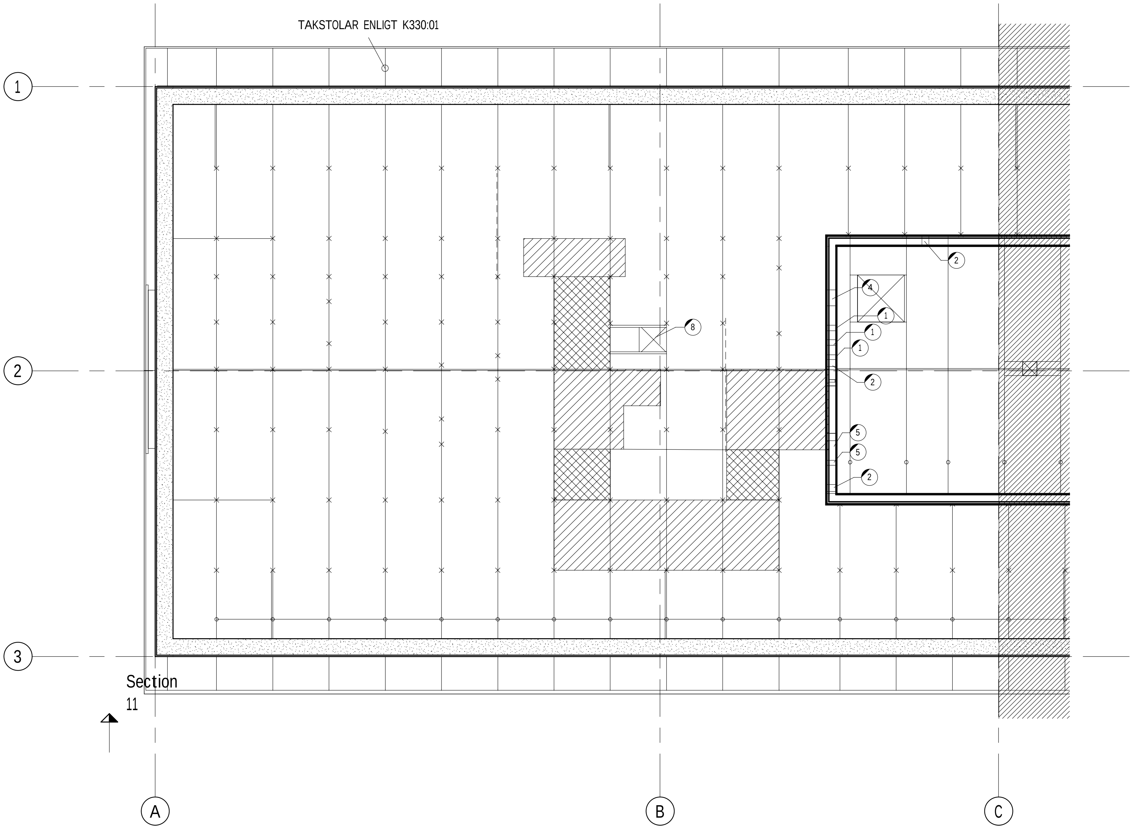
PLAN 3 FLÅKTRUM - Del 1 1 : 50
